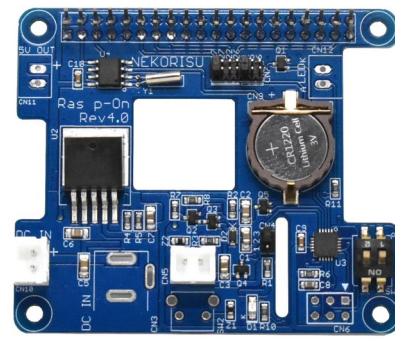
電源入力用コネクタ、スイッチ用コネクタ付き
